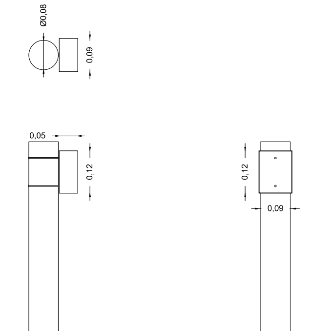
Particolre alloggio dispositivo scala 1:10
